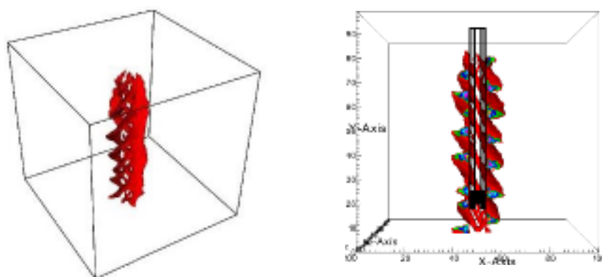
Рисунок 1 – Распределение накопленной неупругой деформации вокруг скважины, (отмасштабировано на максимальное значение неупругой деформации в расчетной области).
