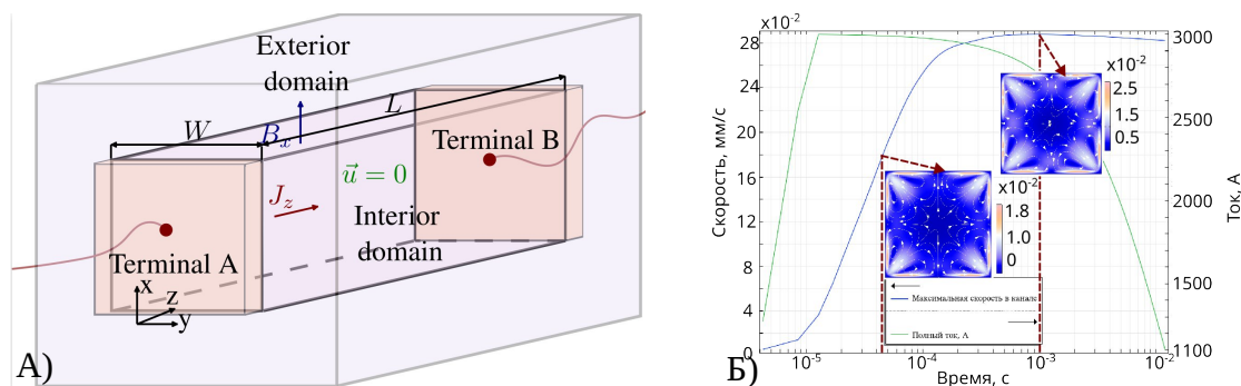
Рис.1. Схематичное представление задачи (А) и зависимость максимальной скорости и тока в канале от времени с пространственным распределением скорости в сечении канала (Б)
