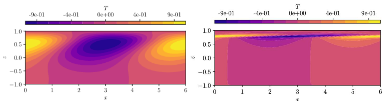
Рисунок 1. Распределение возмущения скаляра, соответствующее наименее устойчивой моде при Ha=50 , Re=25000 , \kappa=0.7 для значений числа Прандтля Pr=10^{-3} (слева) и Pr=1 (справа)
