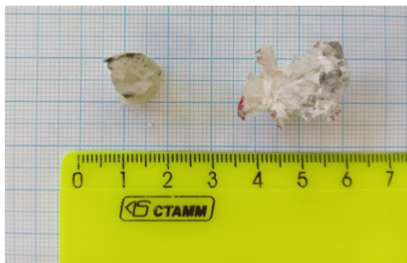
Рисунок 1 – Дефектный образец до и после испытаний
