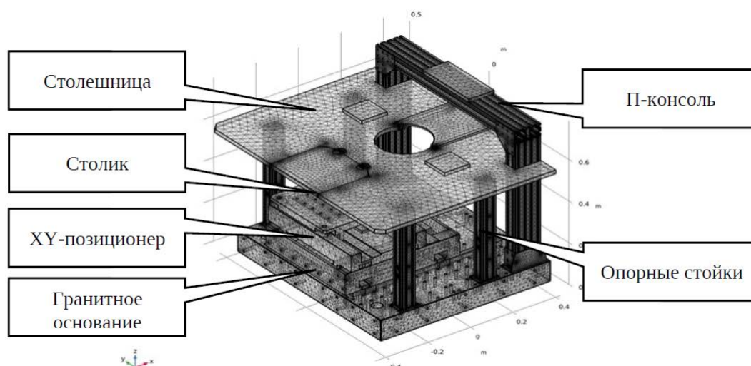
Рис. 1. Схема конечно-элементной сетки и общий вид зондовой станции
