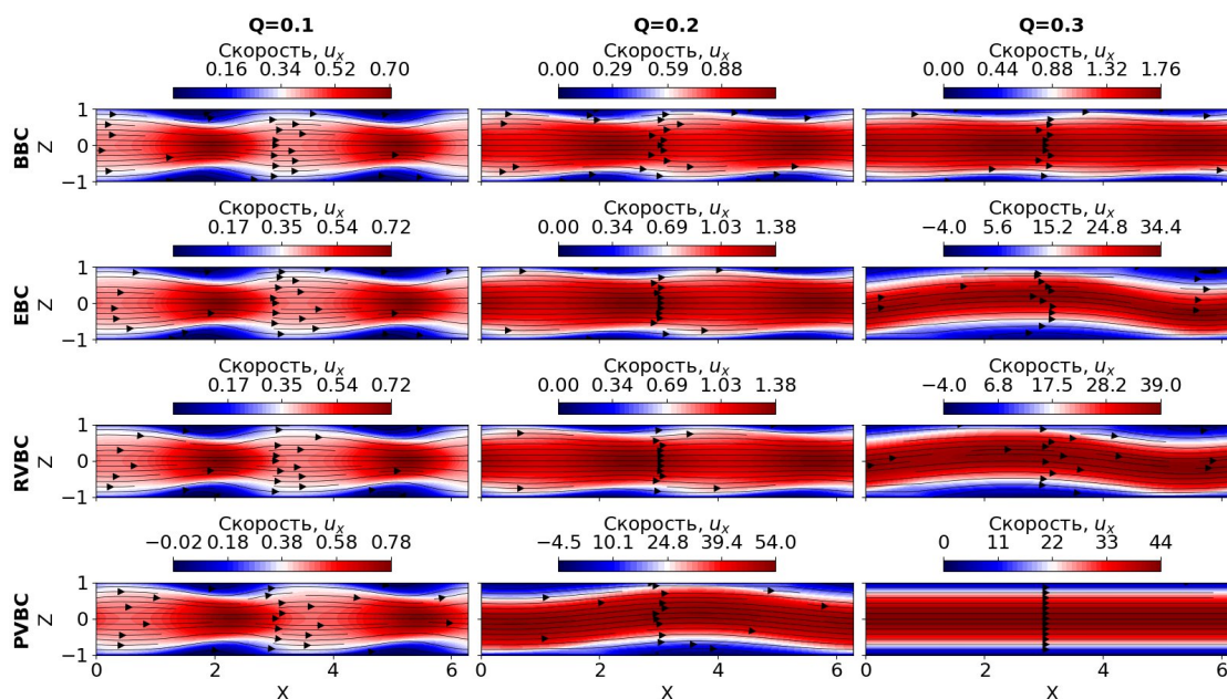
Рисунок 1. Сравнение результатов численного расчета распределений продольной компоненты скорости u_x при использовании в модели ГУ из [1] (BBC), «точных» ГУ с помощью псевдоспектрального метода (EBC), явного разрешения области (RVBC) и псевдовакуумных ГУ (PVBC) для значений Q=0.1-0.3 , соответствующих обратному числу Стюарта.
