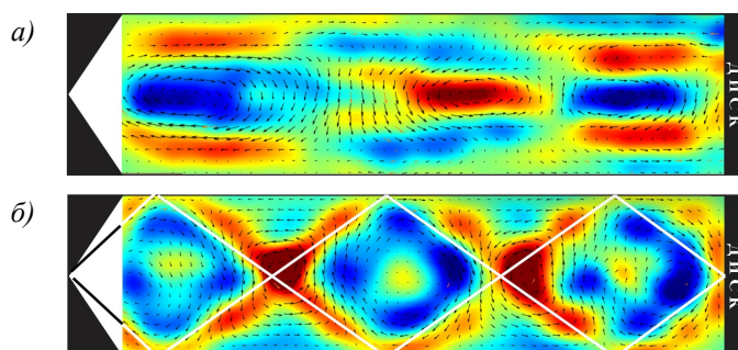
Рис. 1. Мгновенное поле скорости при N = -0.400 (а) и N = -1.263 (б)
