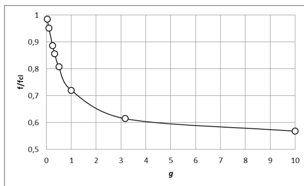
Рис. 1. Зависимость отношений максимальных прогибов для градиентного и классического вариантов теории упругости от величины градиентного параметра
