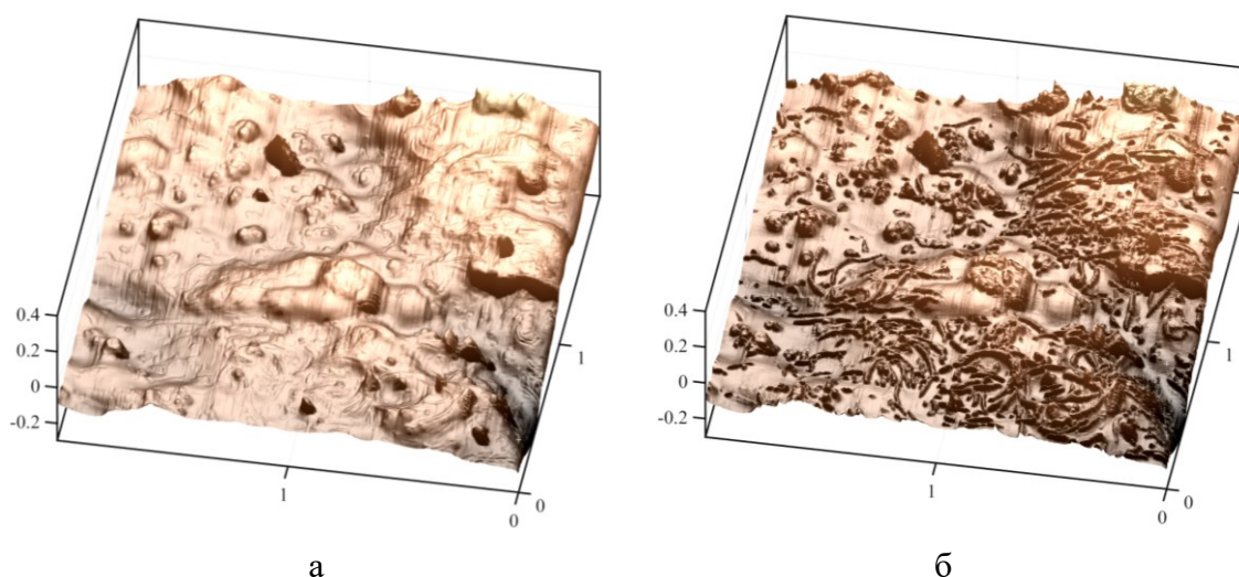
Рис. 1. Иллюстрация метода. (а) – участок поверхности образца (2x2 мкм) по данным АСМ. (б) – трехмерная структура наполнителя в приповерхностном слое, полученная после обработки данных АСМ разработанным методом
