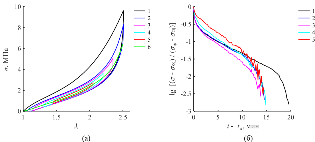
Рис. 2. – Эксперимент со вложенными циклами. Зависимость напряжений от кратности удлинения (а) и зависимость напряжений от времени в процессе релаксации напряжений. Время отсчитывается от момента остановки захватов при максимальной кратности удлинения на данном цикле (б). Цифрами от 1 до 5 отмечены номера циклов. Цифрой 6 отмечена равновесная кривая, полученная сплайном по ключевым точкам
