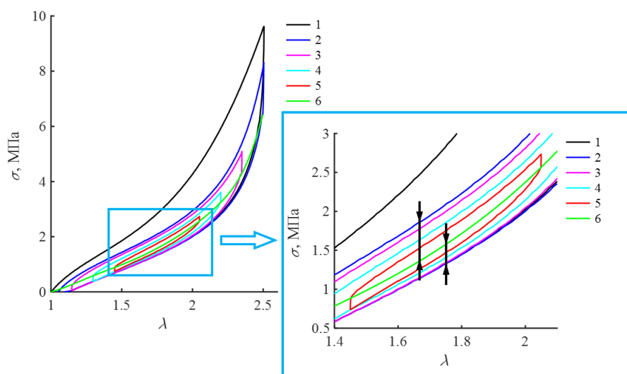
Рис. 4. – Зависимость напряжений от кратности удлинения в эксперименте со вложенными циклами. Цифрами от 1 до 5 указаны номера циклов. Цифрой 6 отмечена равновесная кривая. Стрелками отмечены диссипативные напряжения в установившихся режимах при растяжении образца и при снятии нагрузки
