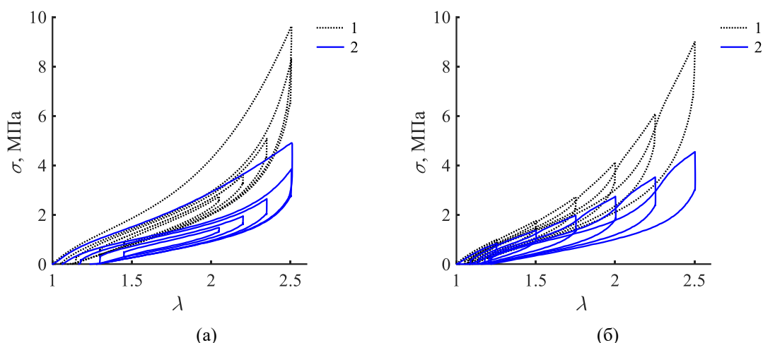
Рис. 2. – Зависимость напряжений от кратностей удлинений в эксперименте со вложенными циклами (а) и в эксперименте с нарастающей амплитудой (б). Наполнителями эластомера являются: 1 – технический углерод, 2 – малослойный графен, полученный из целлюлозы
