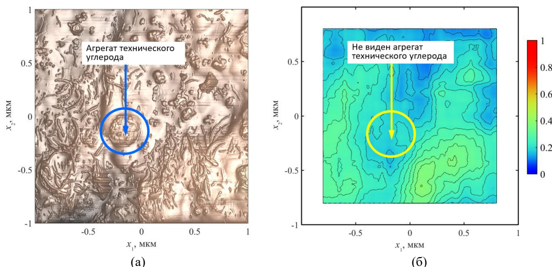
Рис. 3. – С помощью компьютерной обработки эластомер в подповерхностном слое «сделан прозрачным» (а). В результате стали хорошо видны нанотрубки в подповерхностном слое. На рисунке (б) показана, определенная по найденным объектам, карта распределения объемной плотности наполнителя на масштабном уровне R=200 нм (б). Использована методика выделения объектов на основе анализа диссипативных потерь
