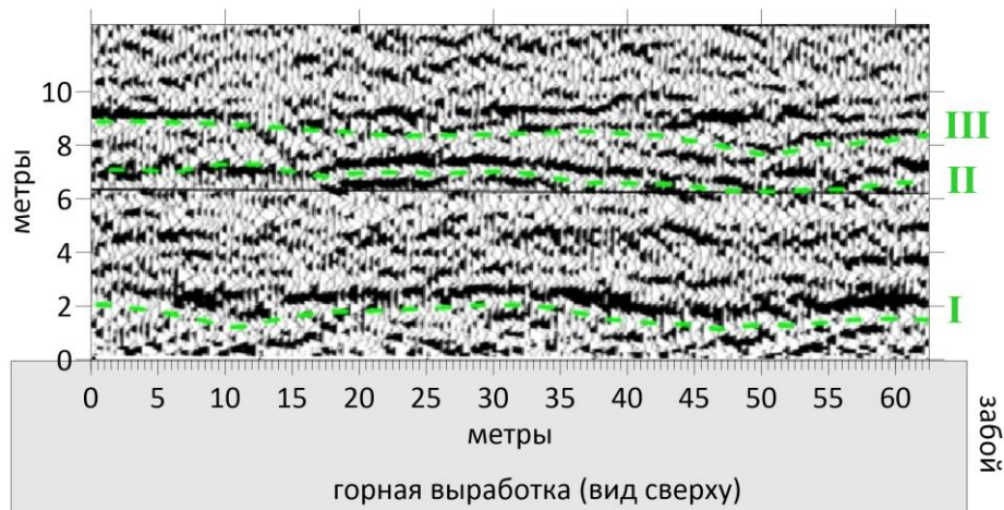
Рис. 1. - Сейсмический разрез Р-волн в горизонтальной плоскости: I – отражение от ближней зоны влияния выработки; II – отражение от дальней зоны влияния выработки; III – отражение от стенки противоположной выработки
