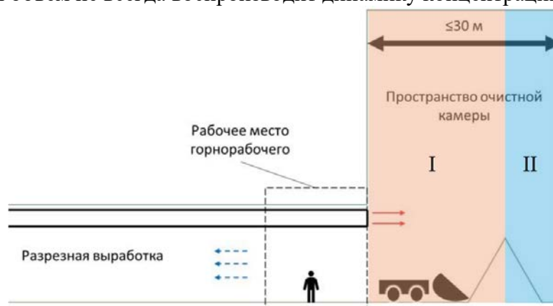
Рис. 1 — Тупиковая очистная камерообразная горная выработка с развалом руды
