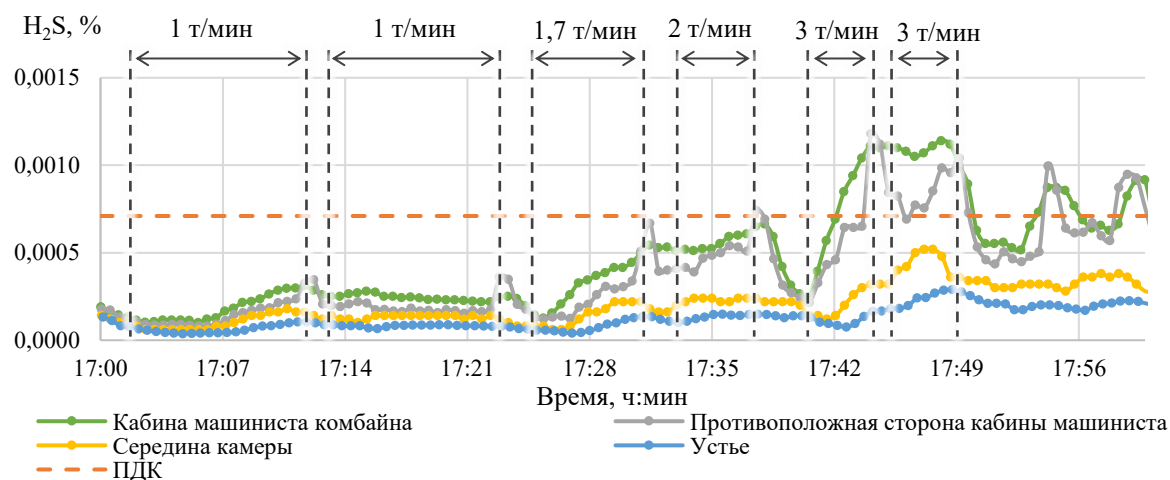
Рис. 1. - Результаты измерений концентрации газа при изменении производительности проходческо-очистного комплекса
