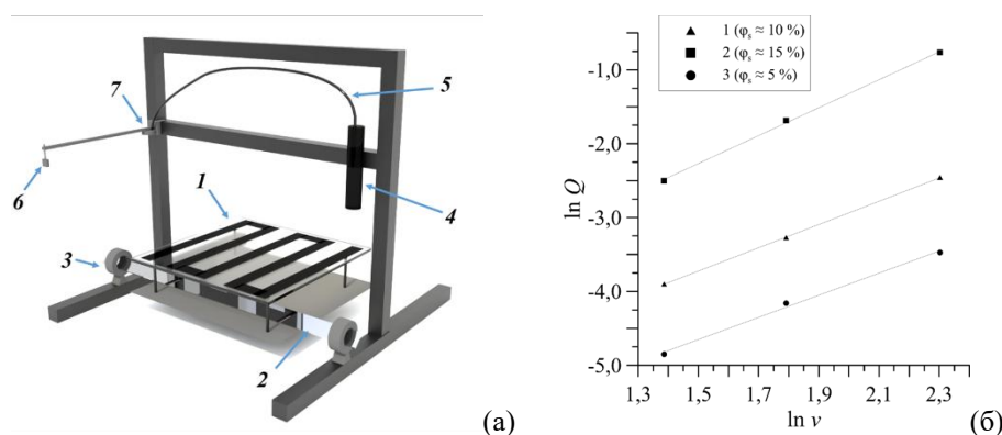
Рис. 1. - Схема лабораторной установки: 1 – стеклянная пластина, 2 – зеркало, 3 – боковые механизмы для регулировки зеркала, 4 – резервуар с магнитной жидкостью, 5 – фторопластовый канал, 6 – зеркало, 7 – датчик, 8 – слой магнитной жидкости (а); зависимость натурального логарифма объемного расхода Q от натурального логарифма скорости движения границы v (б)
