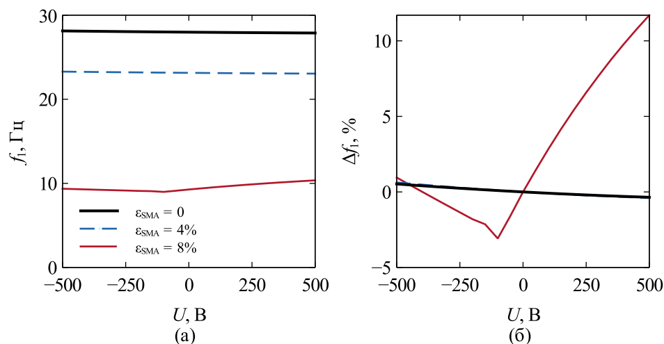
Рис. - Низшая собственная частота пластины (а) и её относительное изменение (б) в зависимости от напряжения U на пьезоэлементе при трёх уровнях \varepsilon_{\text{SMA}}
