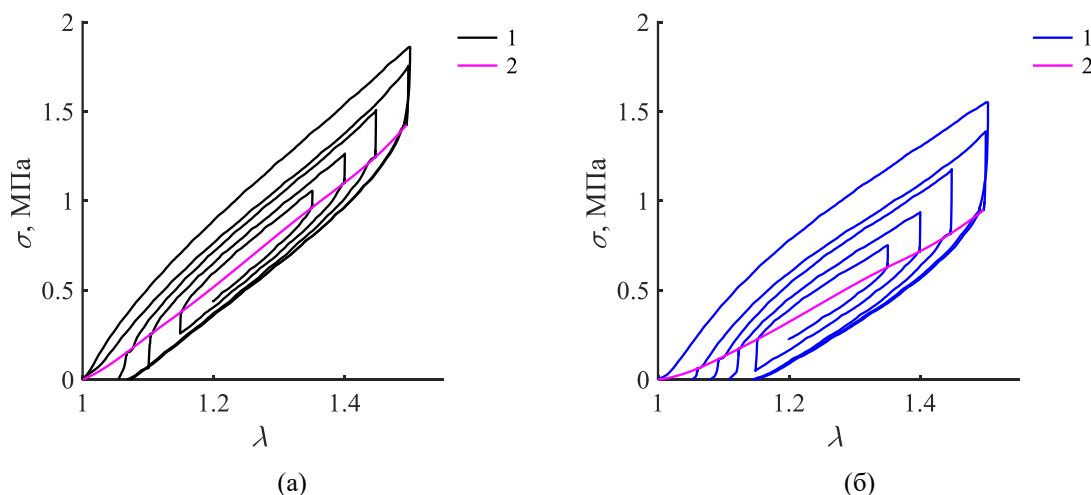
Рис. 3. – Зависимость напряжений от кратностей удлинений в эксперименте со вложенными циклами. Наполнителями эластомера являются: а – технический углерод, б – малослойный графен, полученный из целлюлозы. Цифрой 1 отмечены экспериментальные кривые. Фиолетовыми линиями, отмеченные цифрой 2, показаны равновесные кривые, полученные сплайн-аппроксимацией по ключевым точкам
