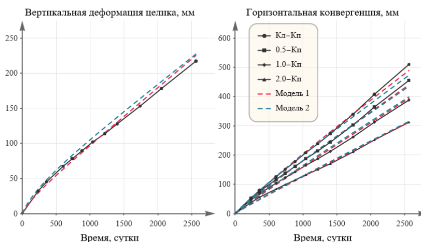
Рис. 1. – Результаты моделирования процесса деформирования камерного сегмента во времени в камере пласта КрII. Обозначения: Кл – контурный левый репер; Кп – контурный правый репер; 0.5–3.0 – глубинные реперы (глубина установки, м), расположенные на левой стороне очистной камеры.
