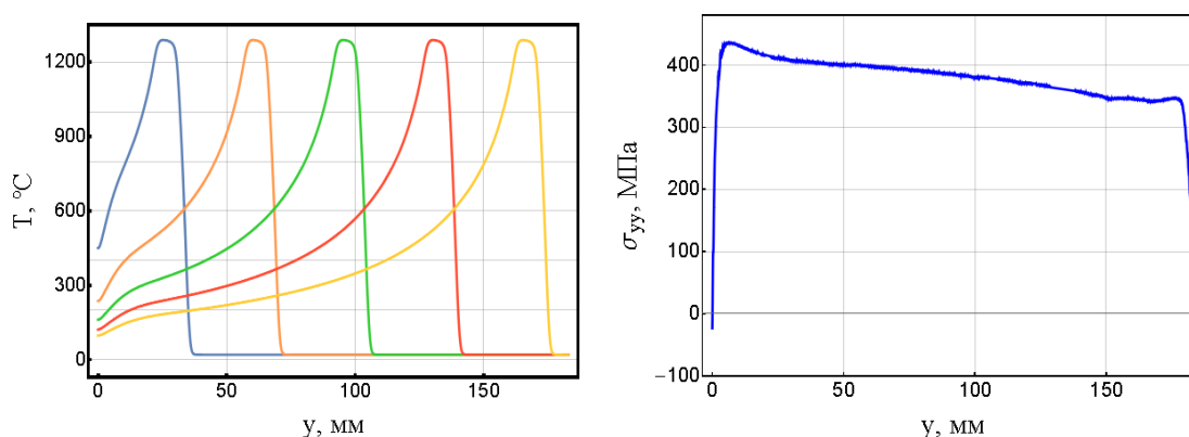
Рис. 3. – Распределения по длине стенки а) температуры в последовательные моменты времени, б) продольной компоненты напряжений
