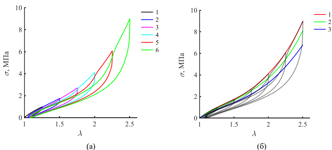
Рис. 3. – Эксперимент с нарастающей амплитудой циклов деформирования. Зависимость напряжений от кратности удлинения с первого по шестой циклы (а) и те же данные с вычисленными по сплайнам кривыми (б), соединяющими точки при максимальных значениях деформаций на цикле для неразмягченного материала (1), размягченного материала (2), размягченного материала при равновесном деформировании (3)
