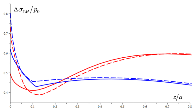
Рис. 1. – Зависимость амплитудных значений напряжений фон Мизеса от глубины при наличии растягивающих (а) и сжимающих (б) остаточных напряжений при наличии покрытия (гладкие линии) и без него (пунктирные линии); \nu = 0,3 , \delta = 0,1a/R
