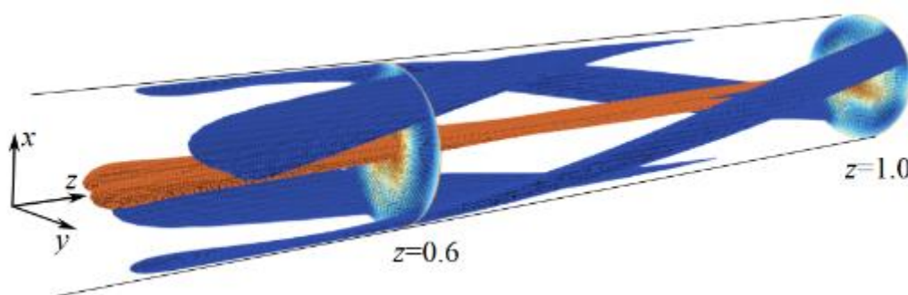
Рис. 2. - Иллюстрация изоповерхности поля тангенциальной скорости при B_2 = 0.15 Тл, B_3 = 0.10 Тл. Синим цветом показано вращение против часовой стрелки, красным - по часовой
