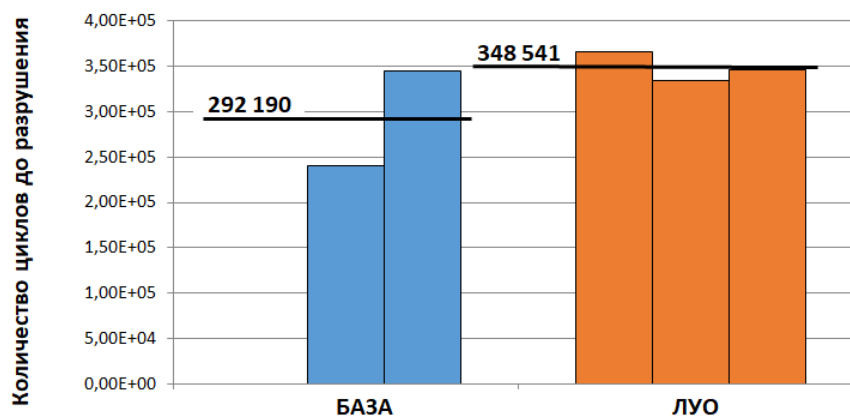
Рис. 3. – Диаграмма усталостной долговечности базовых образцов и образцов после ЛУО
