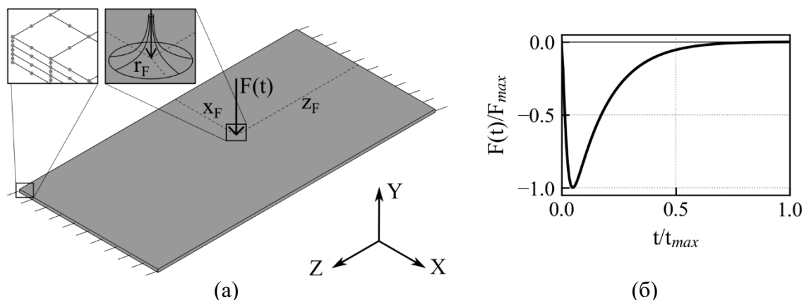
Рис. 1. – Тонкостенная пластина под действием локальной импульсной нагрузки: общий вид модельной задачи (а); форма прикладываемого импульсного воздействия (б)
