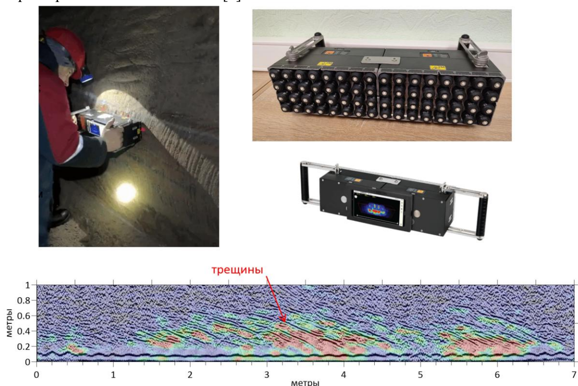
Рис. 2. - Результаты опробования ультразвукового томографа A1040 MIRA 3D PRO при просвечивании целика
