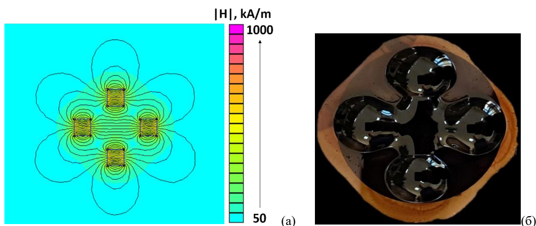
Рис. 1. – Картина распределения модуля напряженности магнитного поля |H| вблизи рассматриваемой системы из кубических магнитов (а); форма свободной поверхности магнитной жидкости вблизи рассматриваемой системы из кубических магнитов (б)
