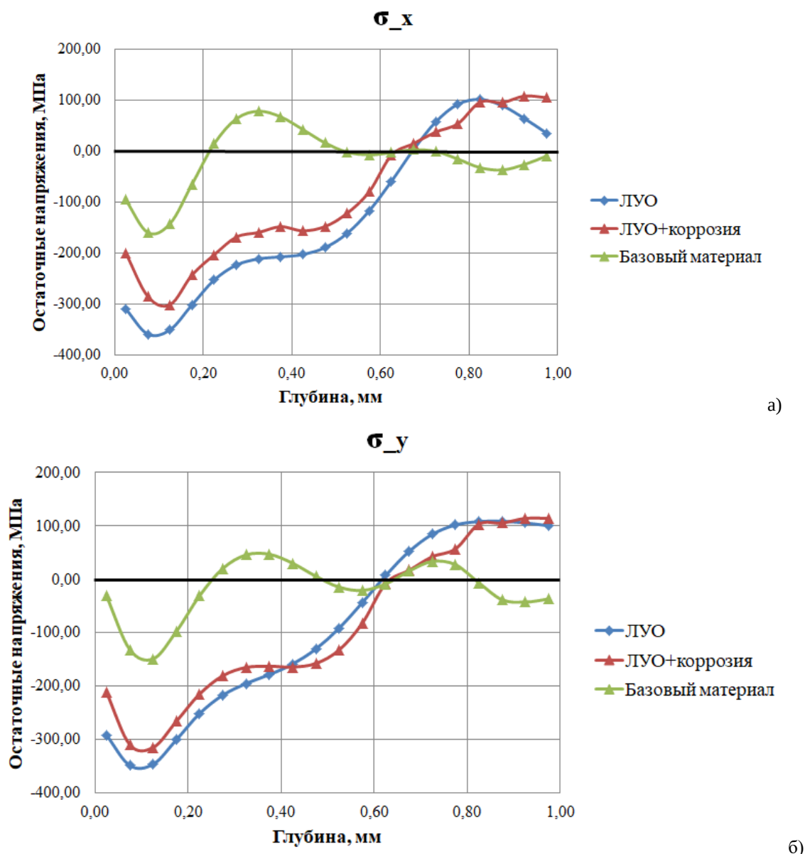
Рис. 1. - Профили компонентов \sigma_x (а) и \sigma_y (б) остаточных напряжений по глубине на базовом материале и после различных типов воздействия на образец: ЛУО и ЛУО+коррозия
