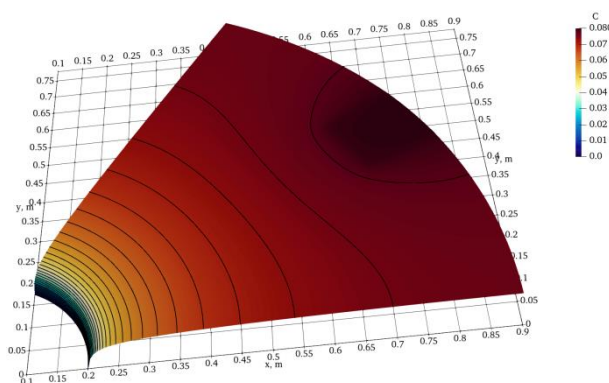
Рис. 2. - Стационарное распределение концентрации кремния на высоте 21 см для конфигурации с четырьмя тиглями
