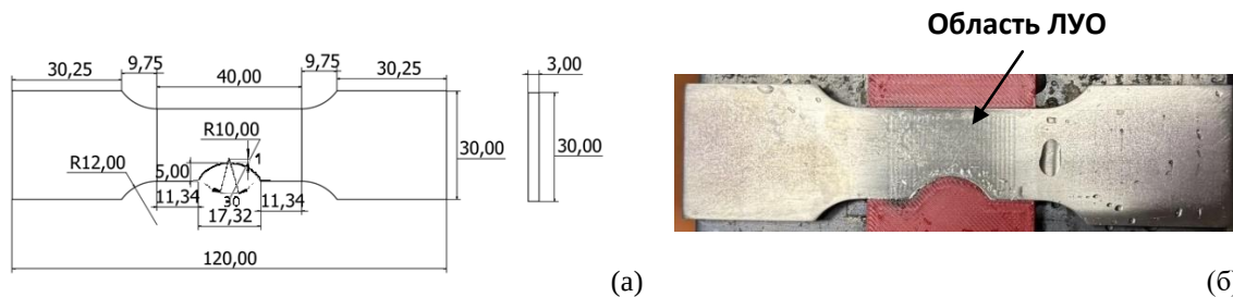
Рис. 1. – Геометрия образцов из титанового сплава ВТ6, изготовленных аддитивным методом (а); фото образца после ЛУО (б)
