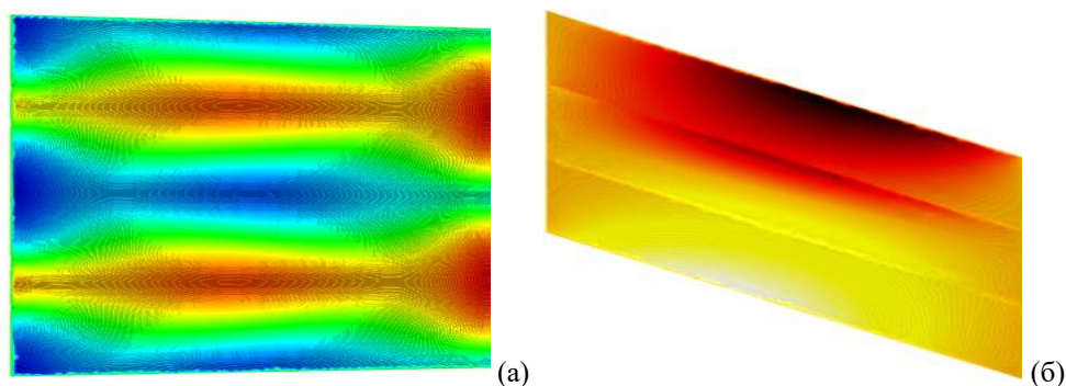
Рис. 2. – Изолинии скорости в крыле складки: вертикальная составляющая скорости вдоль среднего слоя при высоких проницаемостях слоев (а); горизонтальная составляющая скорости в плоскости, перпендикулярной боковым границам слоя, при невысоких близких проницаемостях слоев (б)
