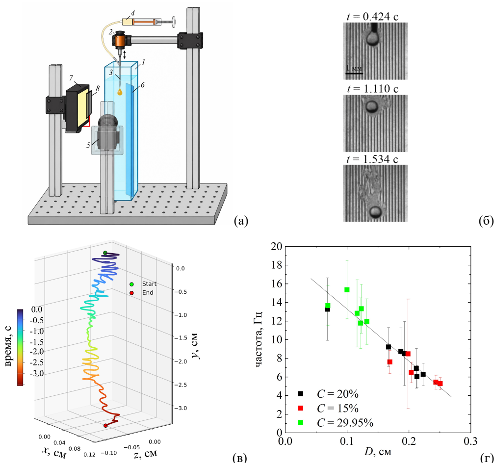
Рис. 1. – Экспериментальная установка (а); визуализация эволюции осаждения капли трехкомпонентной смеси с массовой долей спирта в смеси 29.95% (б); восстановленная трехмерная траектория капли, изображенной на рисунке 1б (в); зависимость средней частоты поперечных колебаний капли от ее диаметра для различного состава смеси (г)
