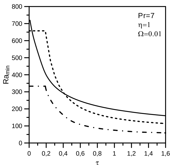
Рисунок 1. Границы устойчивости на плоскости параметров минимальное критическое число Релея – число Деборы. Штриховая линия – в отсутствие модуляции силы тяжести, сплошная и штрихпунктирная линии – при наличии модуляции с параметрами, указанными на рисунке; сплошная линия – аналитическое решение, штрихпунктирная линия – решение, полученное численно методом Рунге-Кутты.
