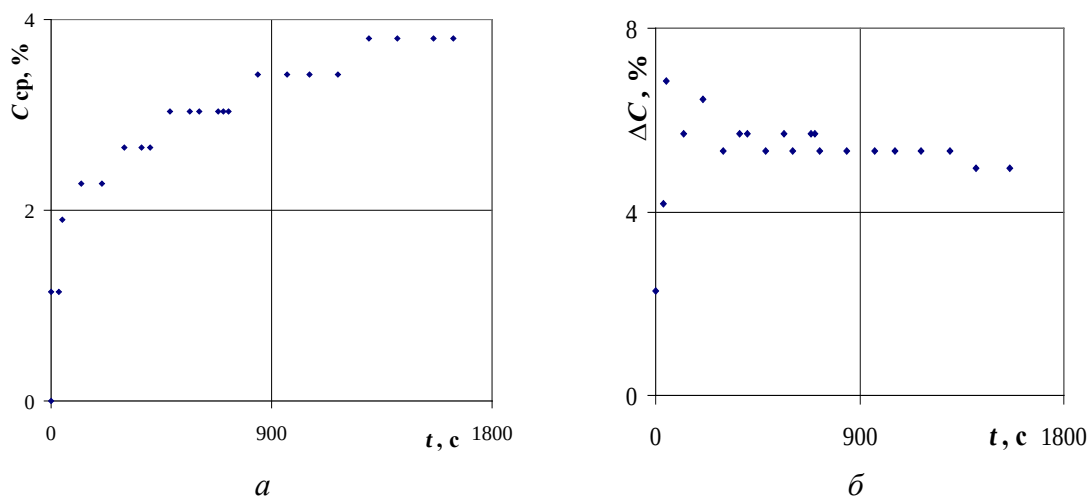
Рис. 4. Зависимости от времени средней концентрации в объеме окружающего раствора ПАВ на уровне экватора капли (а) и перепада концентрации ПАВ между полюсами капли на момент «вспышки» конвекции Марангони (б).
