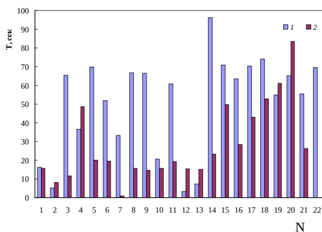
Рис. 2. Зависимости капиллярной (1) и гравитационной (2) составляющих периода осцилляций от порядкового номера периода для капли с пузырьком в растворе этилового спирта с исходной концентрацией C_{01} = 4.2 моль/л.
