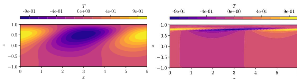
Рисунок 1. Поля возмущений температуры, соответствующие наименее устойчивой моде при Na=50 , Re=25000 , \kappa=0.7 для значений числа Прандтля Pr=10^{-3} (слева) и Pr=1 (справа)
