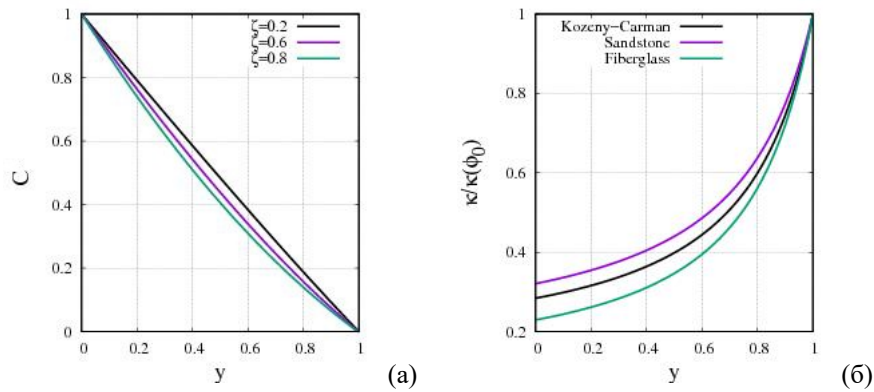
Рис. 1. – Зависимости приведенной концентрации мобильной компоненты ( C – приведена к перепаду концентраций между границами слоя, рис. (а)) и приведенной проницаемости ( \kappa приведена к \kappa(\phi_0) – проницаемости чистой среды, рис. (б)) от координаты поперек слоя ( y ). Кривые на рис. (а) соответствуют различным значениям параметра закупорки, который характеризует максимально возможную степень закупорки среды ( 0 < \zeta < 1 ), кривые рис. (б) соответствуют различным моделям закупорки так: \sigma = 0, \eta = 1, \kappa(\phi_0) = 0.178\gamma – стандартный Козени-Карман, \sigma = 0.425, \eta = 0.226, \kappa(\phi_0) = 0.055\gamma – песчаник (Sandstone [4]), \sigma = 1.74, \eta = 0.003, \kappa(\phi_0) = 0.013\gamma – стекловолокно (Fiberglass [4]).
