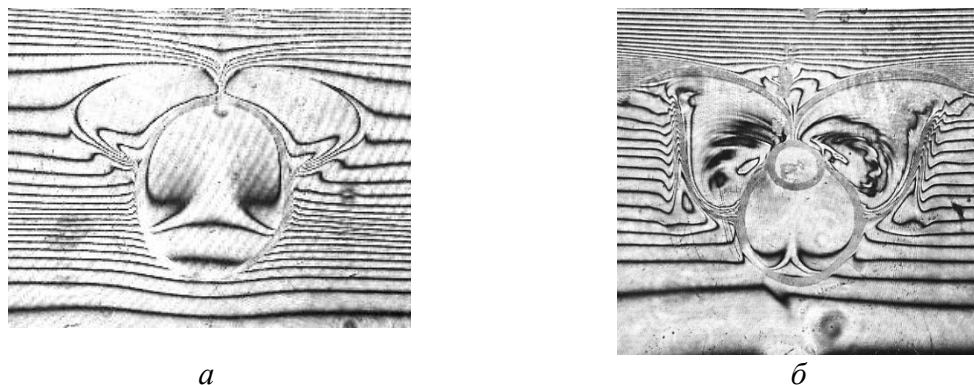
Рис. 3. Интерферограммы полей концентрации этилового спирта на момент «вспышки» конвекции Марангони для случая капля с D_0 = мм и пузырька с d_0 = мм (а) и с D_0 = мм и пузырька с d_0 = мм (б). Время с начала опыта t = с
