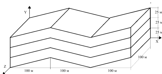
Рис. 1. – Модель геологической складки, имитирующей совокупность антиклинали и синклинали
