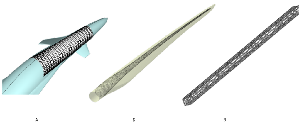
Рис. 1. - Расчетные МКЭ модели конструкции: а) носового отсека делового СПС б) лопасти ветрогенератора в) горизонтальной балки строительного сооружения.
