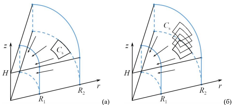
Рис. 1. - Схематическое изображение системы в трехмерной постановке с одним (а) и несколькими (б) тиглями. Стрелками изображен сходящийся поток паров кремния
