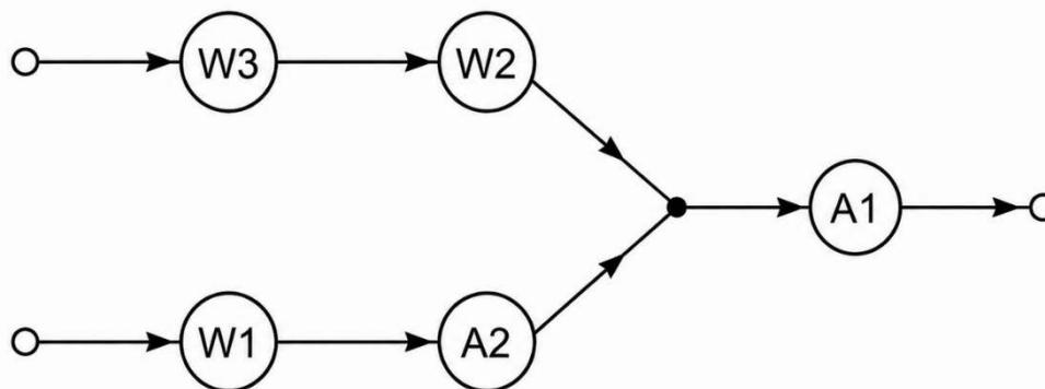
Рис. 1. - Вентиляционная сеть с параллельным соединением ветвей
