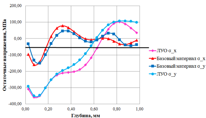
Рис. 2. – Зависимость компонентов остаточных напряжений \sigma_x и \sigma_y от глубины сверления отверстия в базовом материале и в области ЛУО
