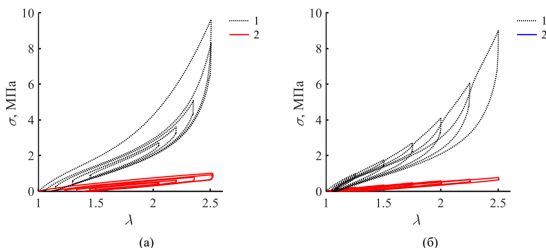
Рис. 1. – Зависимость напряжений от кратностей удлинений в эксперименте со вложенными циклами (а) и в эксперименте с нарастающей амплитудой (б). Цифрами отмечены: 1 – эластомер, наполненный техническим углеродом, 2 – эластомер без наполнителя
