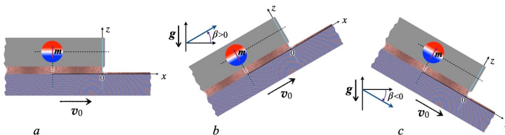
Рис. 1. – Схемы вариантов сканирования плоской поверхности с использованием акустического МЖ-контакта; (а) – случай, рассмотренный в работе [1], (b) – движение датчика вниз по поверхности изделия, (с) – движение вверх. В выполненном расчёте рассматривается только тот край контактного пятна, с которого уносится плёнка.
