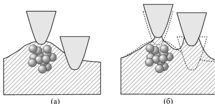
Рис. 1. – Иллюстрации глубины погружения зонда в материал во время его скачка на прямом ходе (а), и количества налипшего на зонд эластомера на обратном ходе (б). В результате отличий в полях напряжений на прямом и обратном ходе появляются диссипативные потери, зависящие от наличия жестких включений под поверхностью образца
