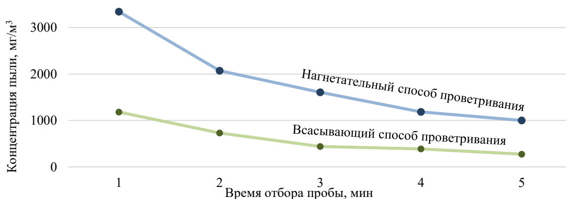
Рис. 2. - Сравнительный график оседания пыли после остановки комбайна
