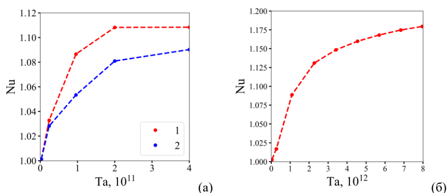
Рис. 1. - Зависимость Nu от Ta для канала переменного диаметра (а) для источника ВМП, расположенного близко к диффузору (1) и близко к середине канала (2); зависимость Nu от Ta для канала переменного диаметра (б)
