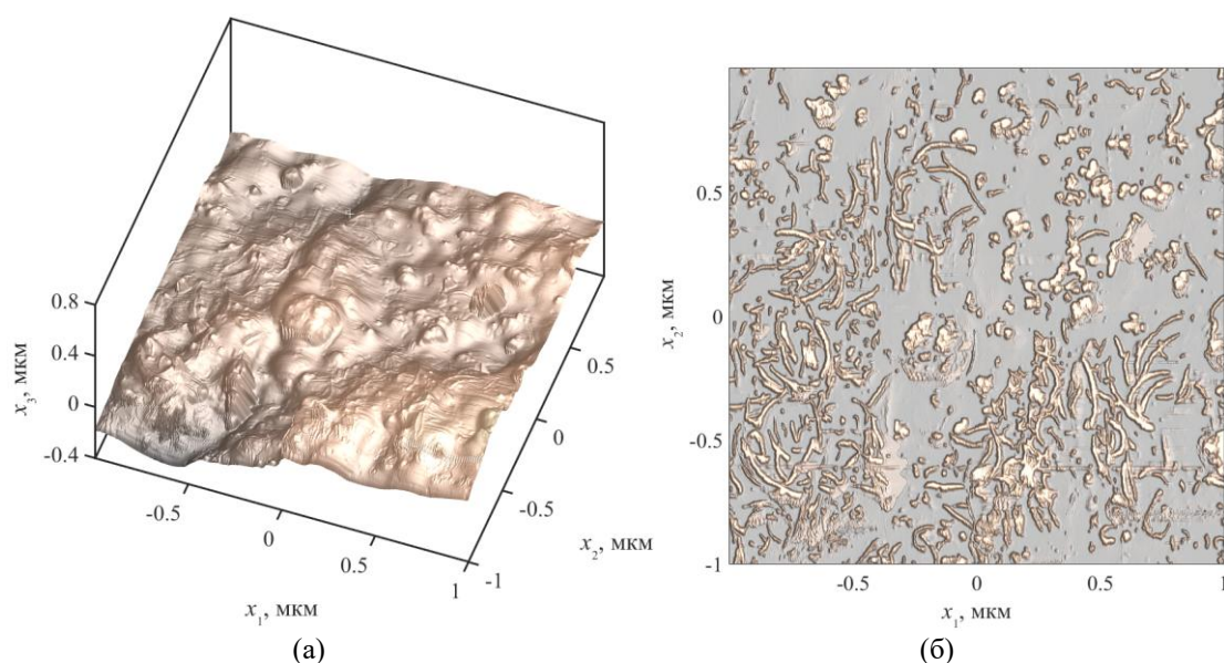
Рис. 2. – Исходная поверхность образца нанокompозита на основе бутадиен-нитрильного каучука, технического углерода и многостенных нанотрубок (а). На рисунке (б) представлена, определенная по новой методике, построенной на основе анализа диссипативных потерь, карта расположения частиц наполнителя в подповерхностном слое образца (б)
