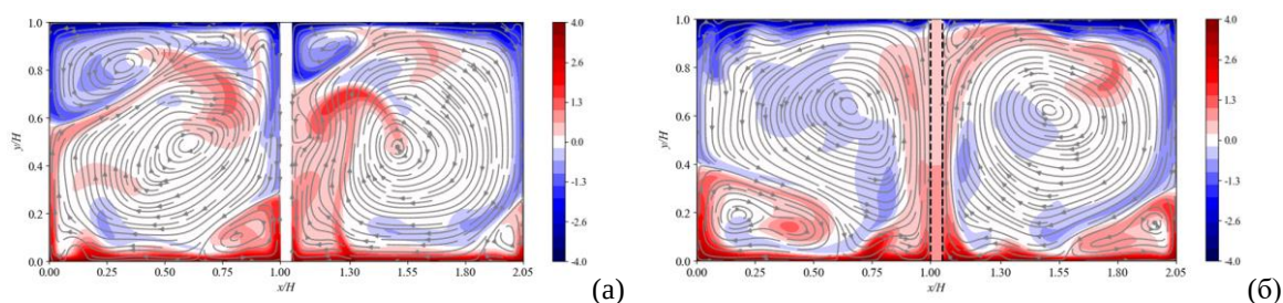
Рис. 2. – Структура КМЦ в случае теплоизолирующей (а) и проводящей (б) границ, цветом показана температура
