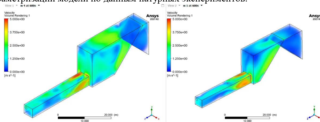
Рис. 2 — Численно рассчитанные распределения скорости в тупиковая очистной камере при различных размерах навала руды
