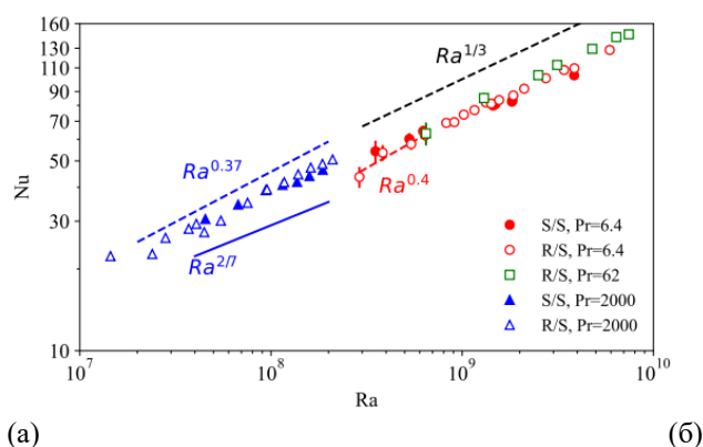
Рис. 1. Сложный рельеф дна (а) и зависимость числа Нуссельта от числа Рэлея для различного рельефа дна и рабочих жидкостей (б).
