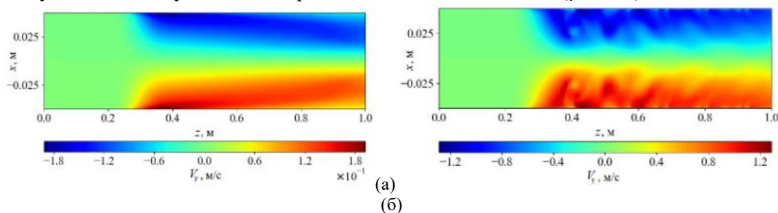
Рис. 1. - Мгновенные поля компоненты скорости V_\varphi в осевом сечении: (а) – B_2 = 0.1 Тл, (б) – B_2 = 0.7 Тл
