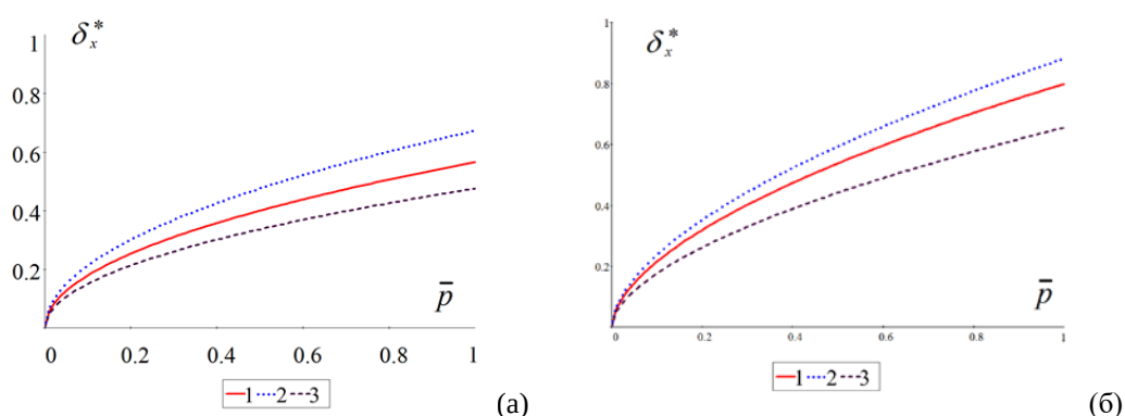
Рис. 2. Зависимость максимального горизонтального сдвига выступов текстуры в начале движения \delta_x^* от номинального давления \bar{p} = P / L_x L_y при n = 1 (а) n = 2 (б) для разных безразмерных амплитуд: A_x/L_x = 0.1 , A_y/L_y = 0.05 (кривая 1); A_x/L_x = 0.1 , A_y/L_y = 0.1 (кривая 2); A_x/L_x = 0.05 , A_y/L_y = 0.05 (кривая 3)
