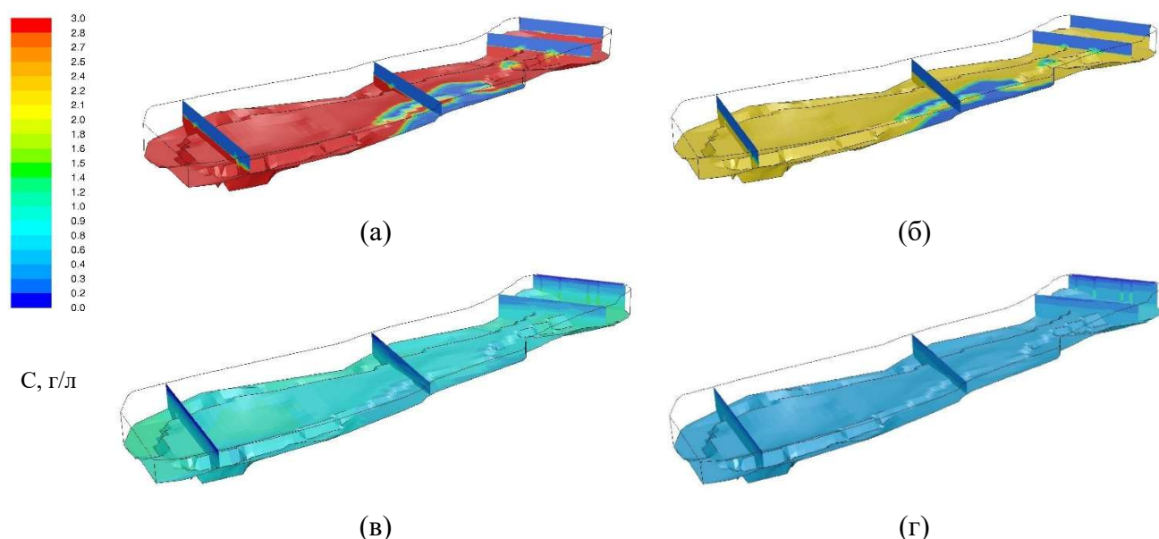
Рис. 1. - Распределения минерализации в створах Верхне - Зырянского водохранилища на дне и в вертикальных сечениях в случае заглубленного сброса воды из водохранилища после, расчетное время (а) - 5 минут, (б) – 12 часов, (в) – двое суток, (г) – пять суток
