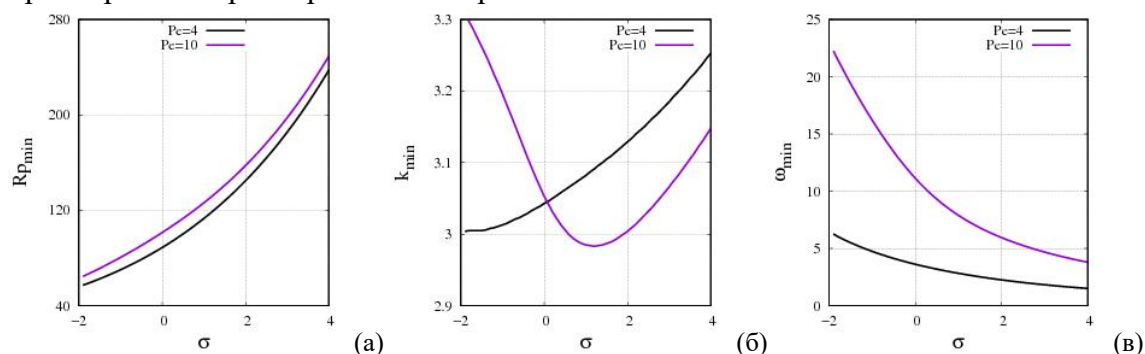
Рис. 3. – Зависимости критического значения числа Релея-Дарси ( Rp_{min} – характеризует силы плавучести, рис. (а)), критического волнового числа ( k_{min} , рис. (б)) и частоты критических возмущений ( \omega_{min} , рис. (в)) от параметра объема зерна ( \sigma ). Кривые соответствуют различным интенсивностям фильтрационного потока ( Pe – число Пекле, отношение скорости фильтрации вдоль слоя в чистой среде к диффузионной скорости).
