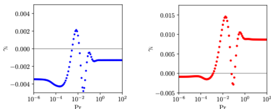
Рисунок 2. Зависимости скорости роста возмущений от числа Прандтля при двух наборах параметров: Na=50 , Re=75000 , \kappa=0.6 (слева) и Na=50 , Re=17500 , \kappa=0.7 (справа)
