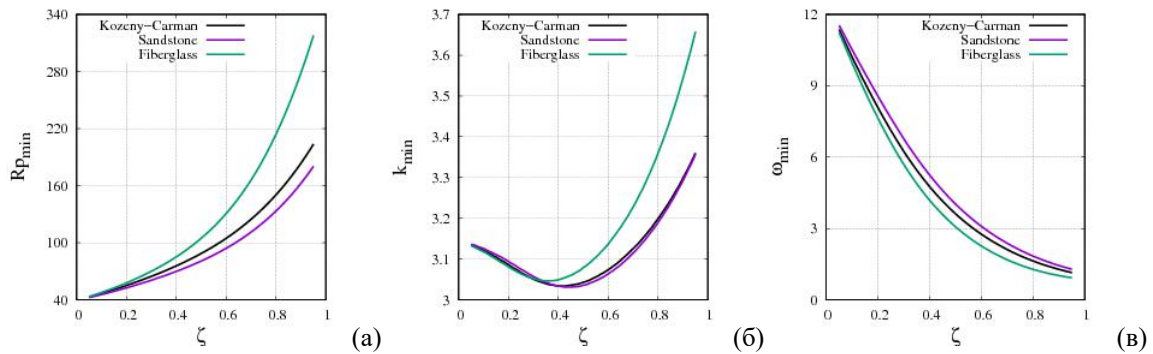
Рис. 2. – Зависимости критического значения числа Релея-Дарси ( Rp_{\min} – характеризует силы плавучести, рис. (а)), критического волнового числа ( k_{\min} , рис. (б)) и частоты критических возмущений ( \omega_{\min} , рис. (в)) от параметра закупорки ( \zeta ). Кривые соответствуют различным моделям закупорки так: \sigma = 0, \eta = 1, \kappa(\phi_0) = 0.178\gamma – стандартный Козени-Карман, \sigma = 0.425, \eta = 0.226, \kappa(\phi_0) = 0.055\gamma – песчаник (Sandstone [4]), \sigma = 1.74, \eta = 0.003, \kappa(\phi_0) = 0.013\gamma – стекловолокно (Fiberglass [4]).
