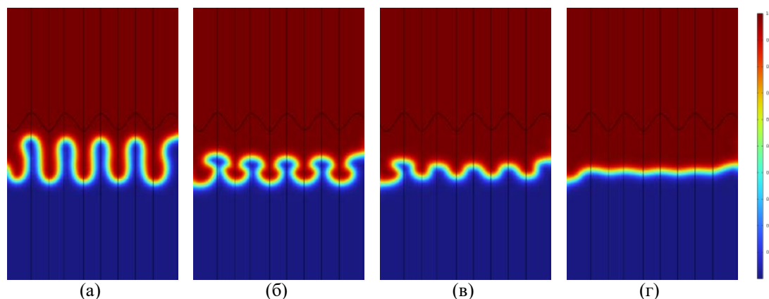
Рис. 1. - Распределение фаз в момент времени 2 с при частоте пульсаций 900 \text{ с}^{-1} и амплитуде осциллирующего перепада давления 50 Па (а), 150 Па (б), 175 Па (в) и 200 Па (г); чёрная кривая – начальное положение фронта
