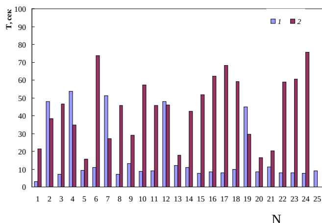
Рис. 1. Зависимости капиллярной (1) и гравитационной (2) составляющих периода осцилляций от порядкового номера периода для капли без пузырька в растворе этилового спирта с исходной концентрацией C_{01} = 4.2 моль/л
