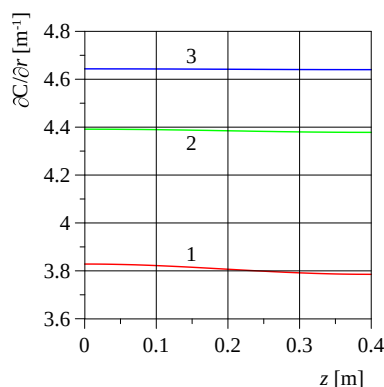
Рис. 3. – Профиль градиента концентрации кремния на поверхности изделия в зависимости от вертикальной координаты. Кривая 1 – конфигурация с одним тиглем. Кривая 2 – конфигурация с двумя тиглями. Кривая 3 – конфигурация с четырьмя тиглями
