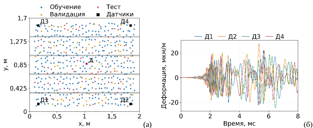
Рис. 1. - Пластина, рёбра, датчики и точки ударов (а). Пример сигналов четырёх датчиков для отмеченного удара (б).
