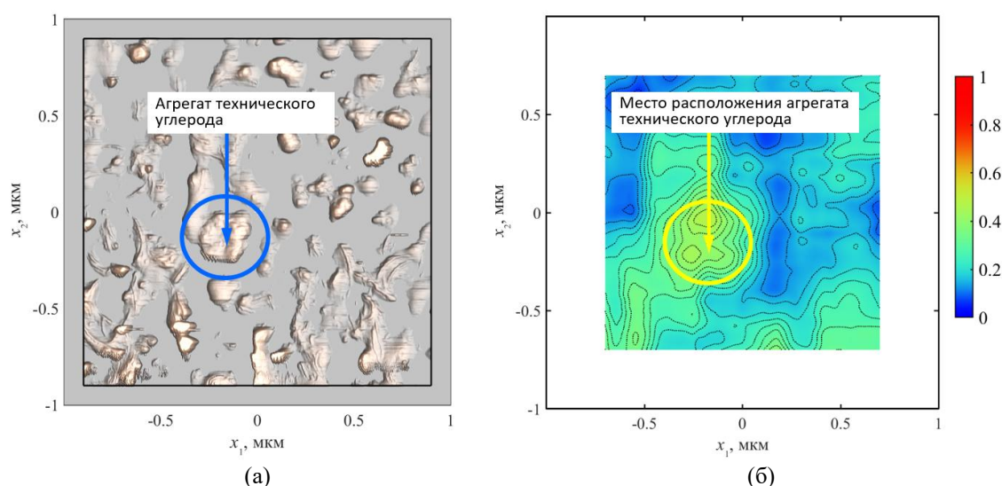
Рис. 4. – Расположение частиц наполнителя, полученное по методике анализа геометрии поверхности образца (а). На изображении не видно нанотрубок. На рисунке (б) показана карта распределения объемной плотности наполнителя на масштабном уровне R=200 нм (б)
